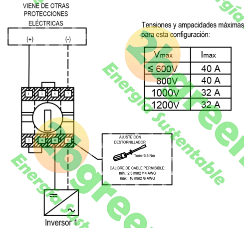
Diagrama 2. Un inversor energizado por un Seccionador SISO-40MD-B Configuración sugerida
