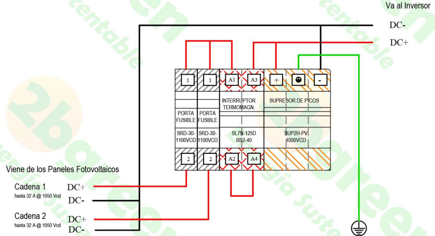
CONEXIÓN SUGERIDA PARA 2 CADENAS, 1 MMPT, 1050 Vcd < V oc (Dos polos en serie, puente en 2 y 4)
