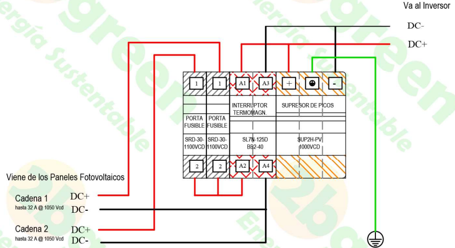
CONEXIÓN SUGERIDA PARA 2 CADENAS, 1 MMPT, 1050 Vcd < V oc (Carga Flotante, sin puente)
